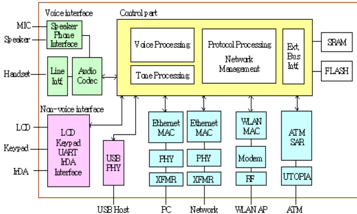
IP 폰 단말의 기능 구성도
